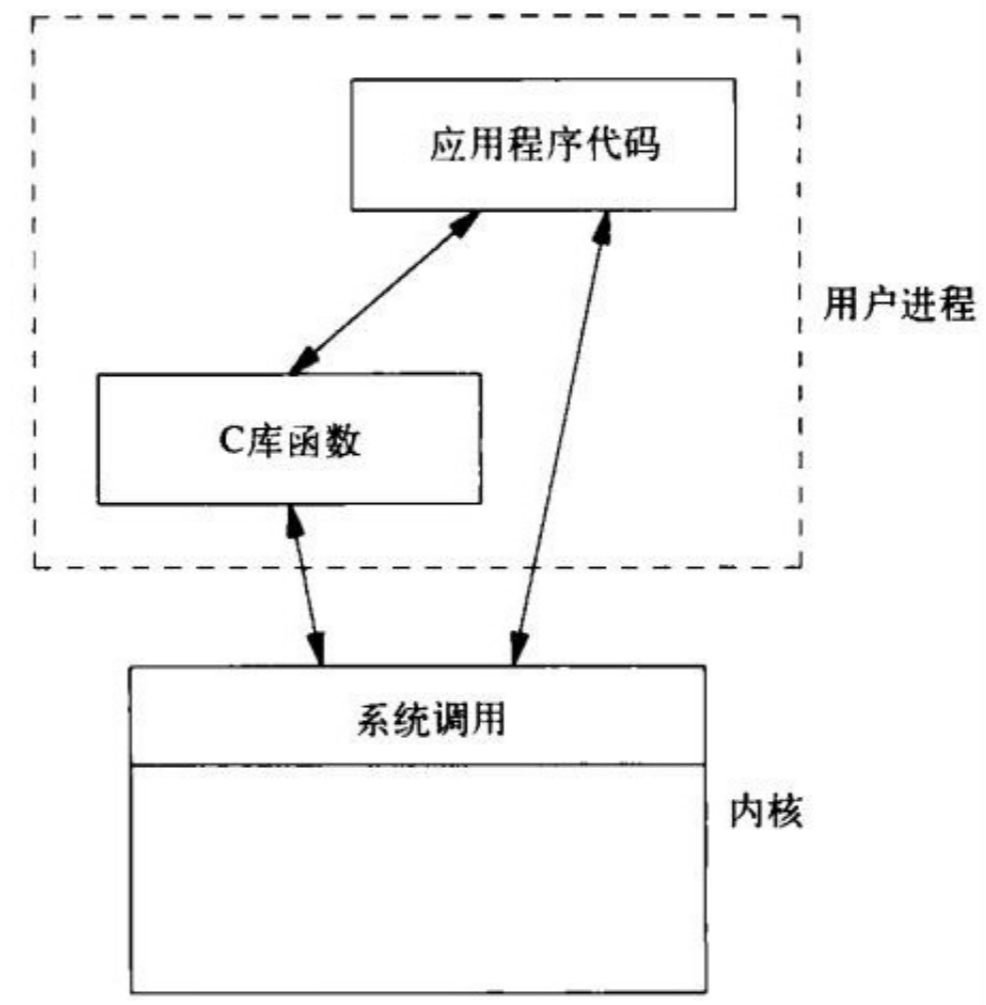
图1-3 C库函数和系统调用之间的差别
