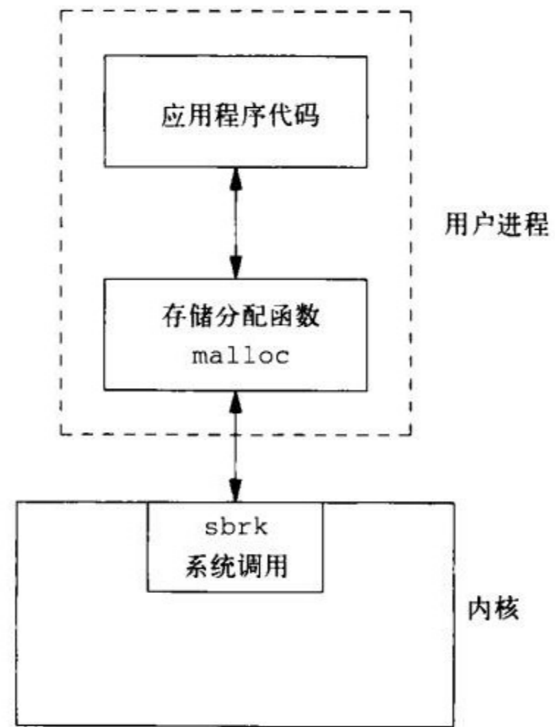
图1-2 malloc函数和sbrk系统调用
